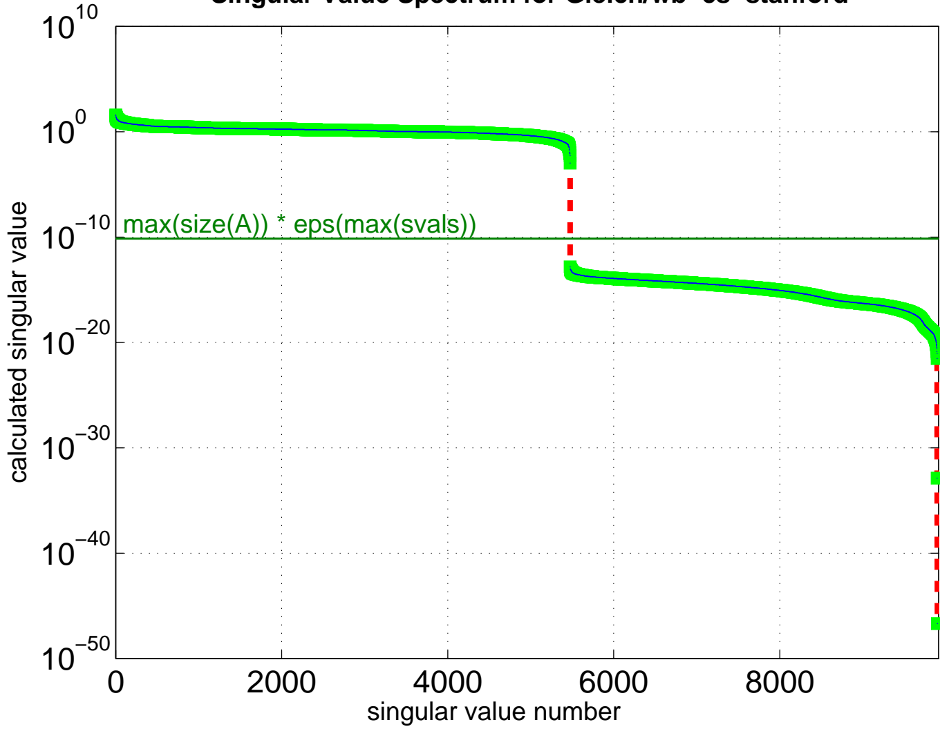
Singular Value Spectrum for Gleich/wb-cs-stanford
