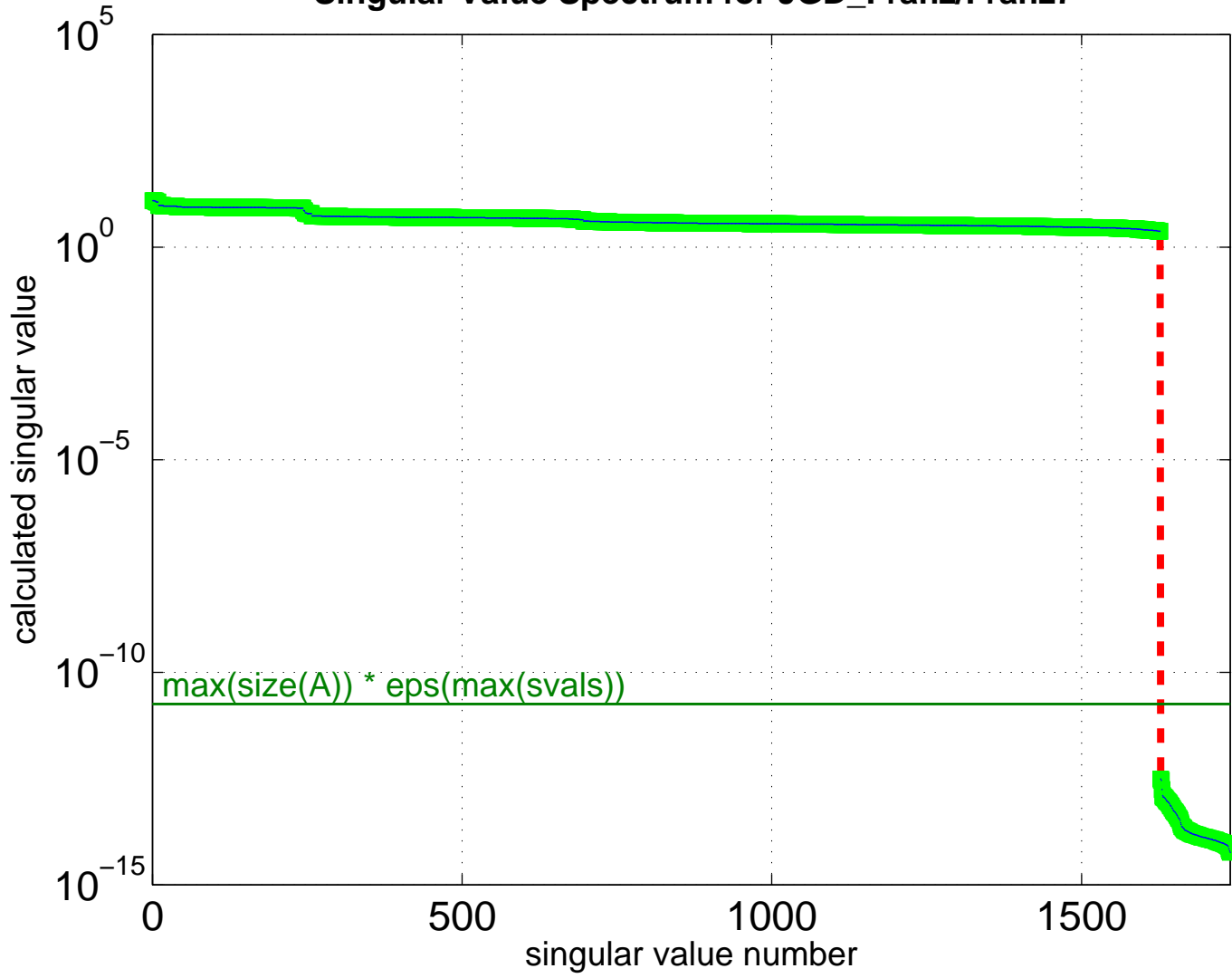
Singular Value Spectrum for JGD_Franz/Franz7
